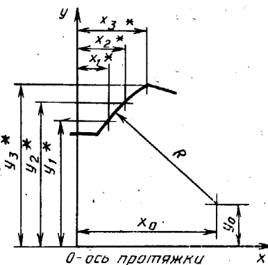
Размеры профиля протяжки на 1-м шлицевом зубе
