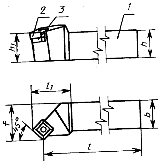
Левый резец
